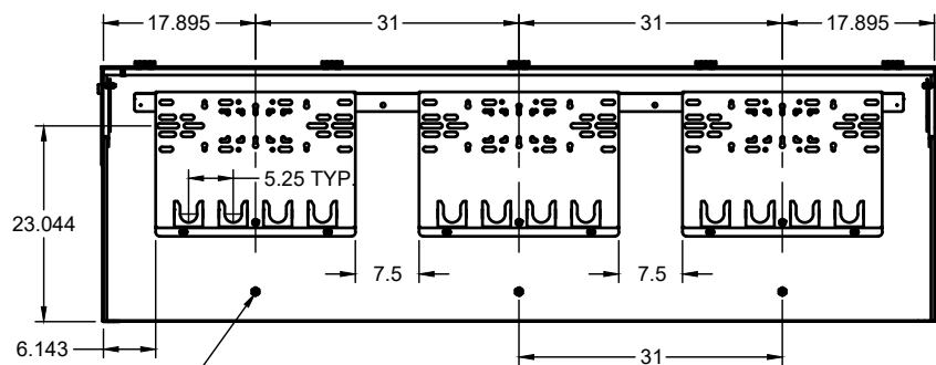
SECTION A-A SCALE 1:25
